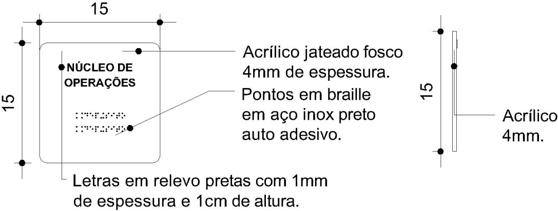
Placa tipo 8 - 15cm x 15cm
